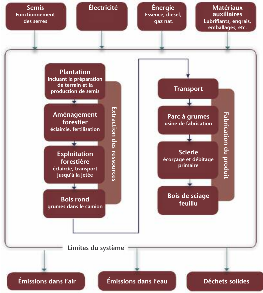
Figure 1 : Limites du système et enchaînement des opérations
